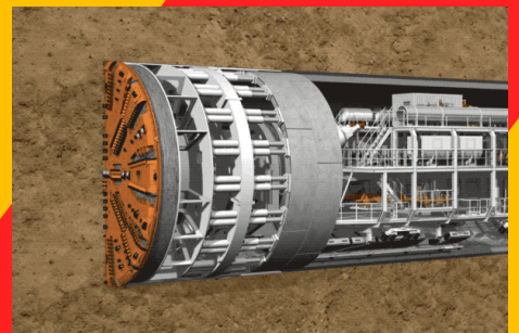
シールド掘削機 地下鉄や上下水道工事で使用される
